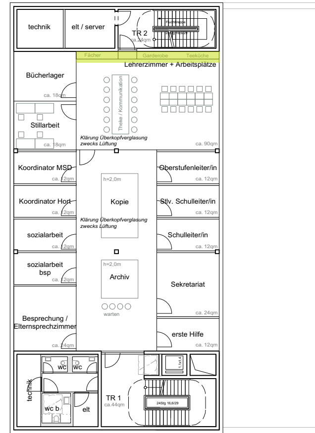
GEMEINSCHAFTSHAUS 2. OG
