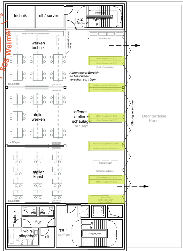
GEMEINSCHAFTSHAUS 1. OG
